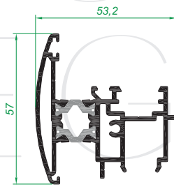
59.3545 Inversor Curvo Hoja
