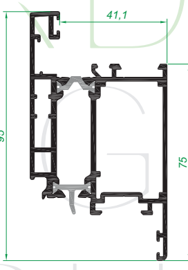
59.2246 Hoja Puerta Recta
