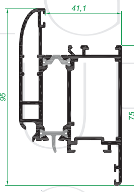
59.2275 Hoja Puerta Curva
